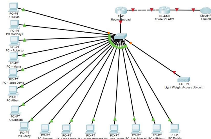
Imagen 12: Topología Red INDUPAL
